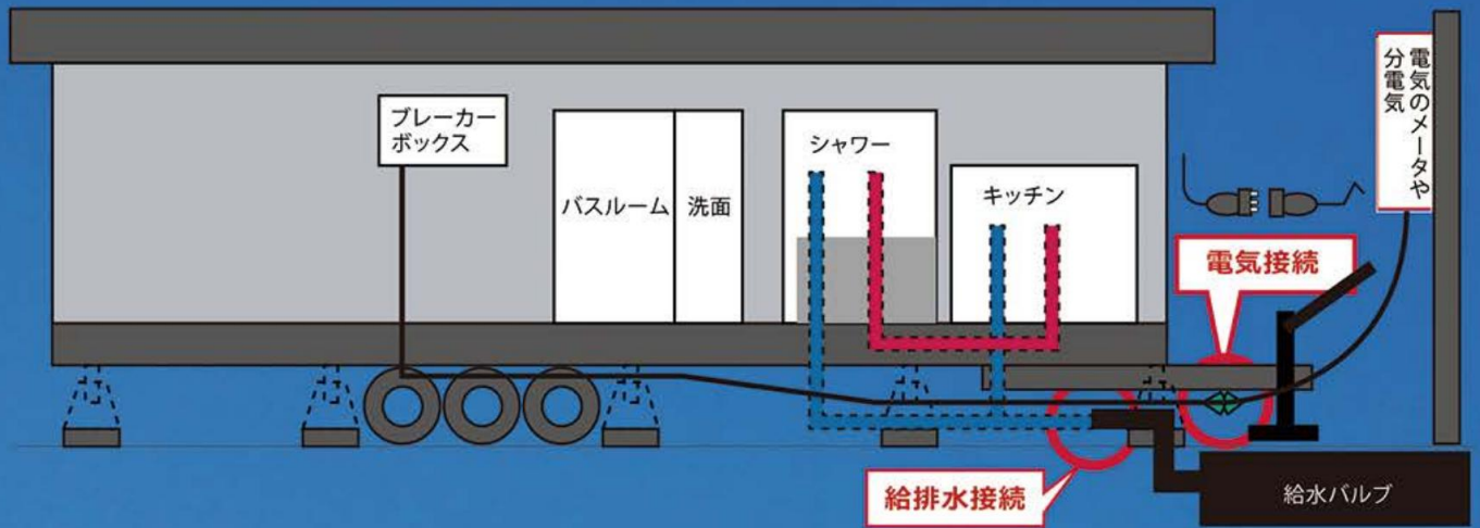
給排水接続の場合
